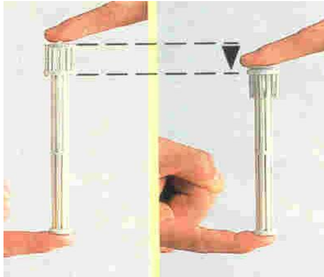
36. pav. Voleliai fiksuojami sustumiant juos per ilgį
